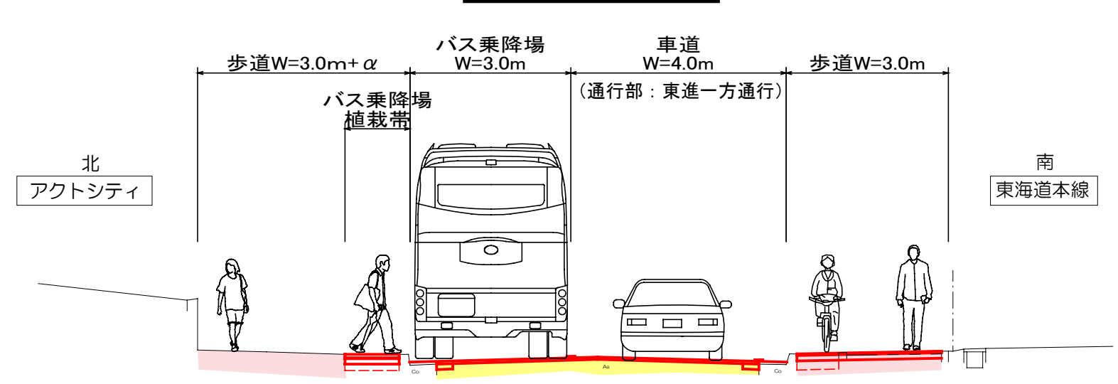
道路標準横断面図
